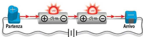
Circuito in serie - 2 segnali luminosi accesi
